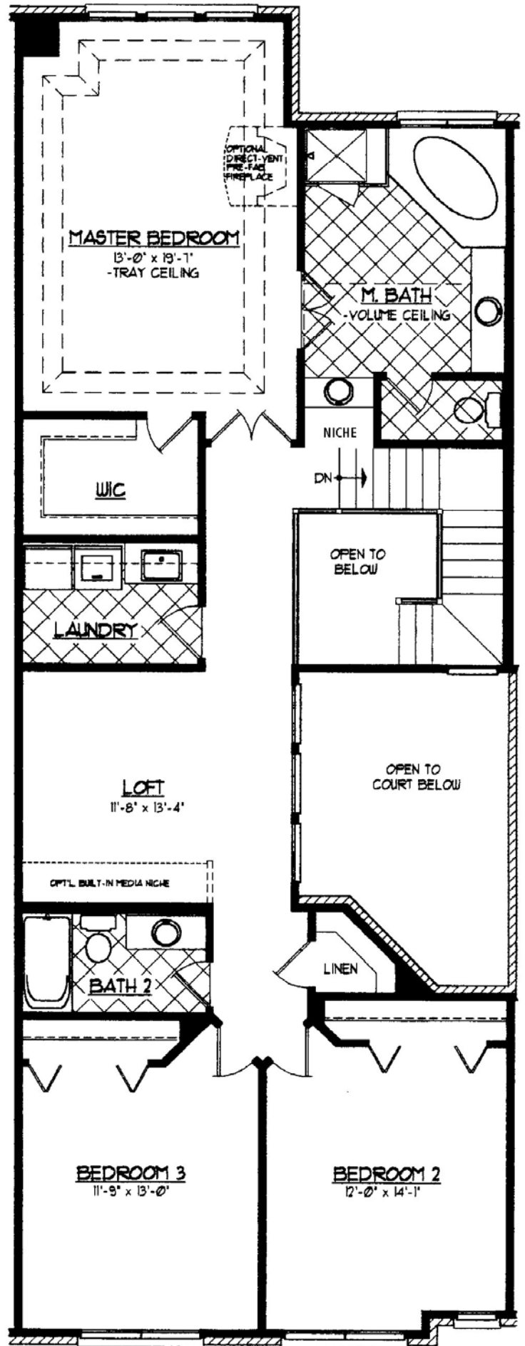
SECOND FLOOR DI AM
